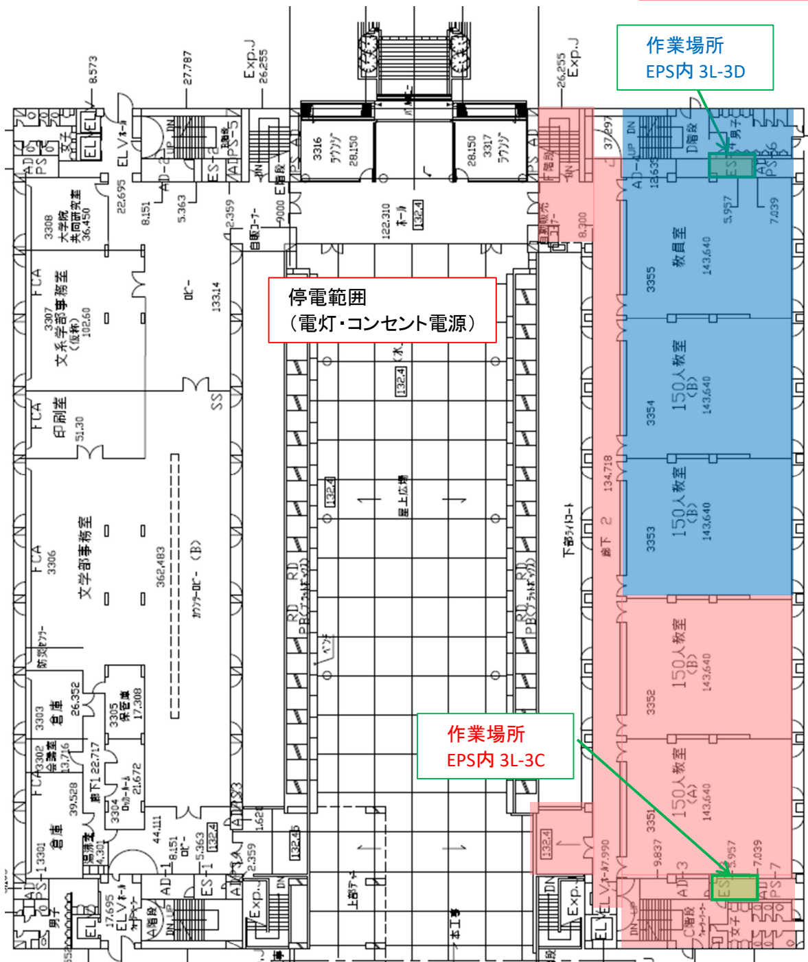
③3階平面図
