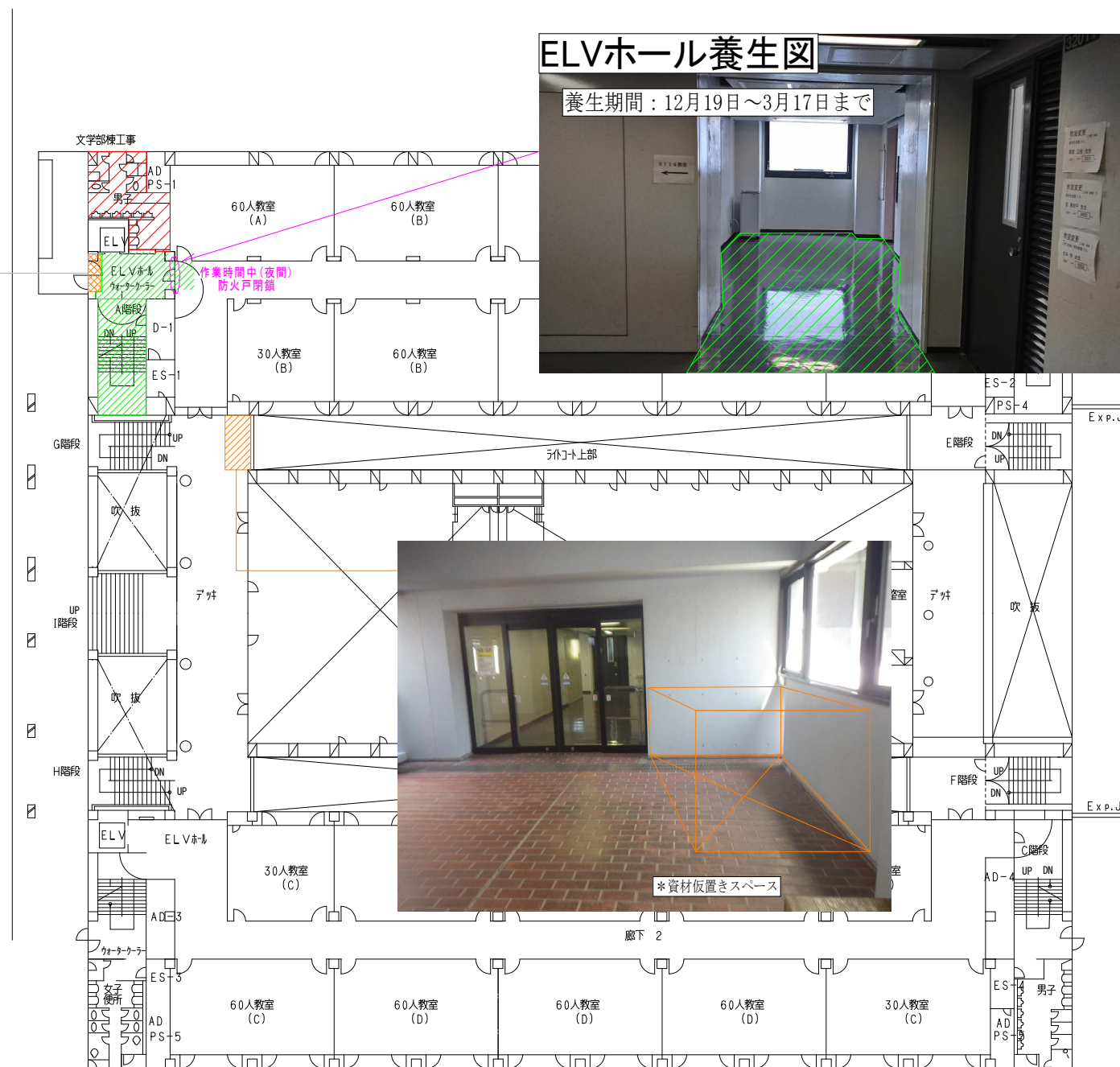
2階平面図
