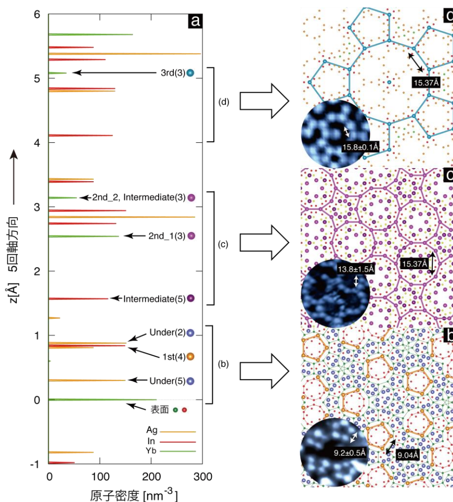
図3(a): 準結晶構造データから求めた基板表面(5回回転対称表面)に垂直な方向の原子密度分布。ここで、Å(オングストローム)は長さの単位で、 1\text{\AA}=10^{-10}\text{m}=0.1\text{nm} (ナノメートル)。 z=0 が表面原子層。図中の矢印は実験で観測された計6原子層(表面に近い側から under 層、第1層、中間層1、第2層、中間層2、第3層)に対応する原子層。カッコ内の数字は図2のクラスタの殻番号。(b-d): 表面から(b) 0 \leq z \leq 0.9\text{\AA} , (c) 1.53\text{\AA} \leq z \leq 3.15\text{\AA} , (d) 5.04\text{\AA} \leq z \leq 5.40\text{\AA} の範囲の原子位置と鉛の吸着量に応じて観測された STM 像(挿入図)。それぞれの STM 像と同じ五角形や10角形が基板準結晶の構造データの中にあることが分かる。
