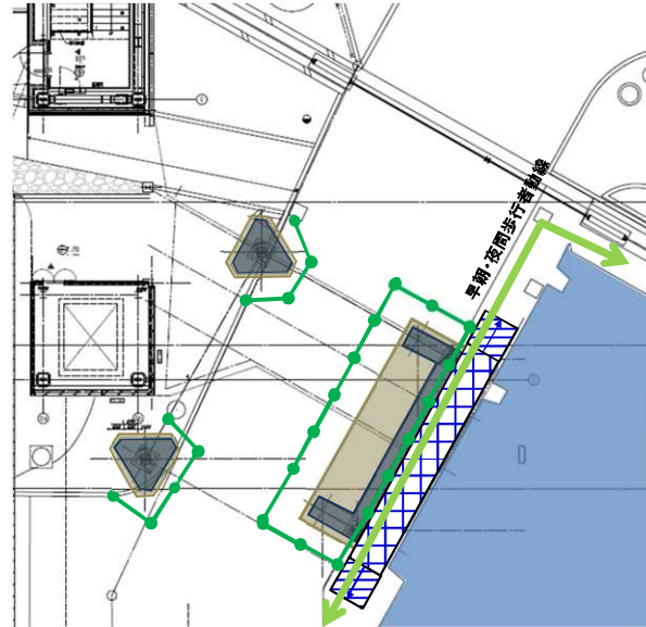
② 北東ブリッジ基礎躯体工事夜間状況 (～8:00、21:00～)
