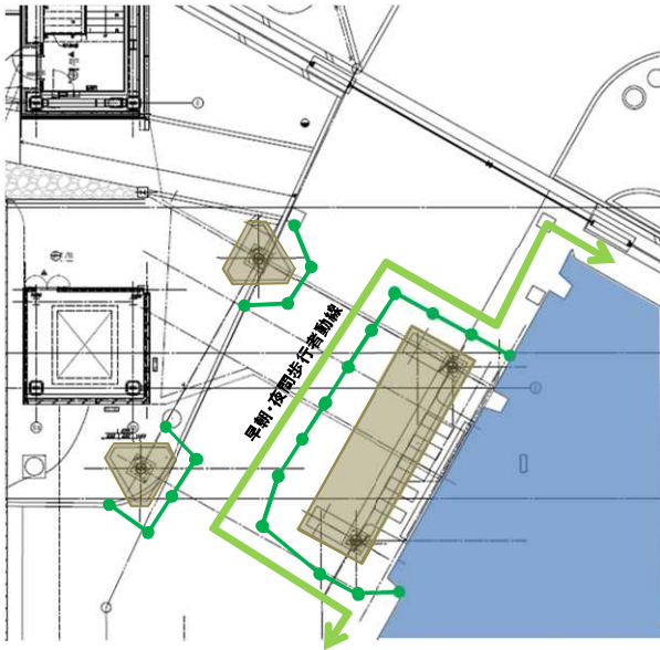
① 北東ブリッジ基礎部分掘削夜間状況 (～8:00、21:00～)
