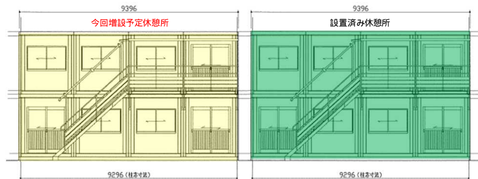
【休憩所立面配置図】
