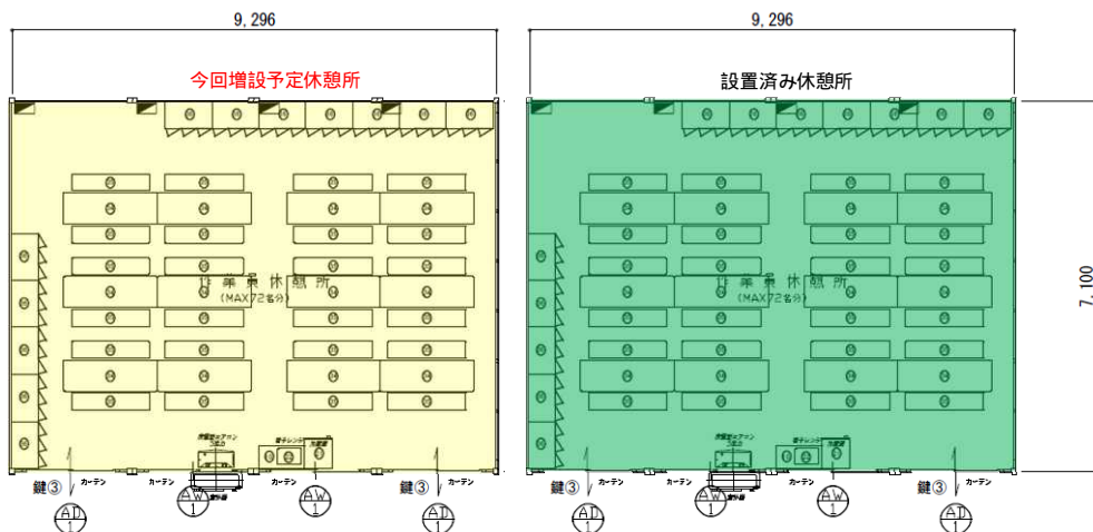
【休憩所平面配置図】
