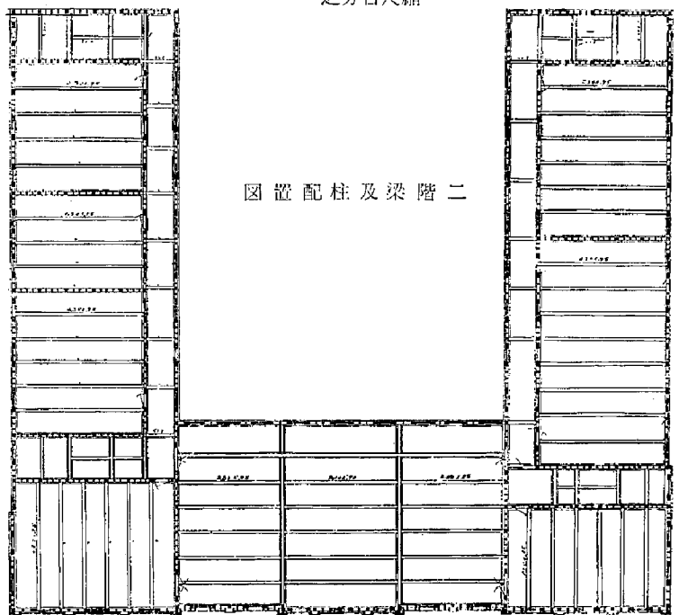
中央大学新舎建築設計圖 縮尺百分之一
