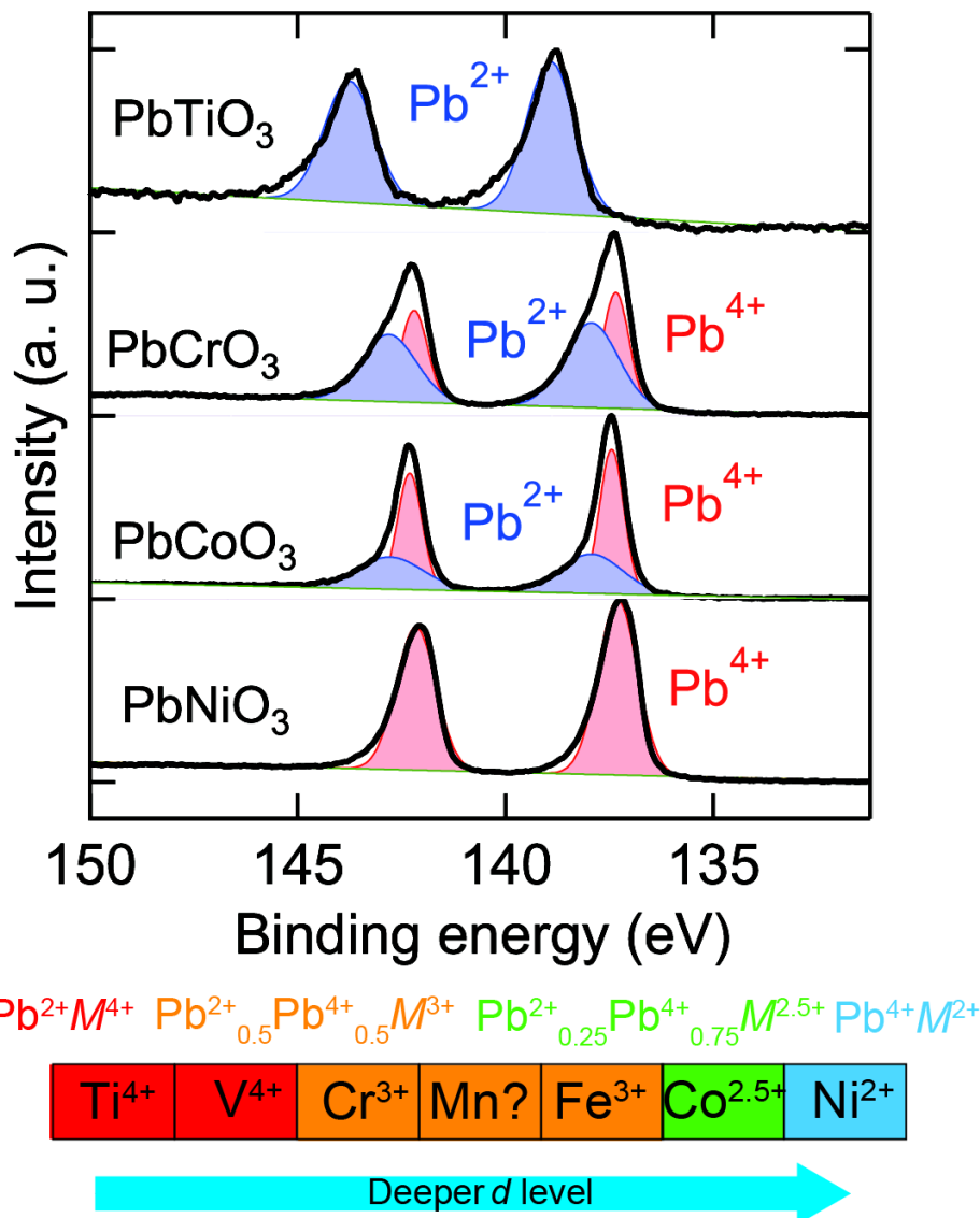
図2 PbMO 3 (M=Ti, Cr, Co, Ni) の硬 X 線光電子分光 (HAXPES) スペクトル
